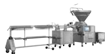
↑ PLSH 217 с функцией навешивания
