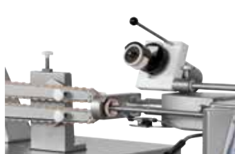
↑ Устройство для вытягивания оболочек ↑ Датчик распознавания конца оболочки
