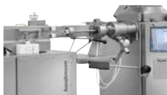
↑ Moedor de embutimento GD 93-3
