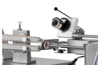
↑ Enfiador de tripa
