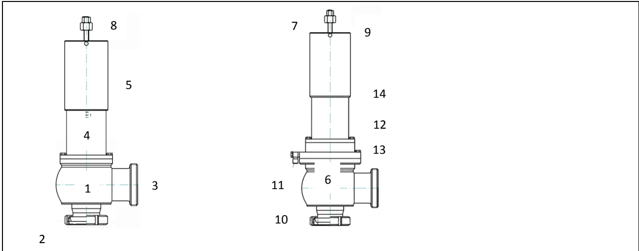
Fig. 1: Type 33502 und 33602
