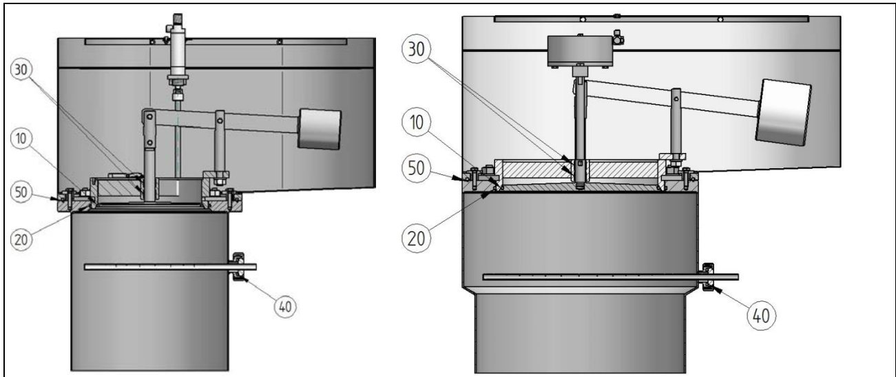
Fig. 6: Tipo 12814 DN 150 – 200
