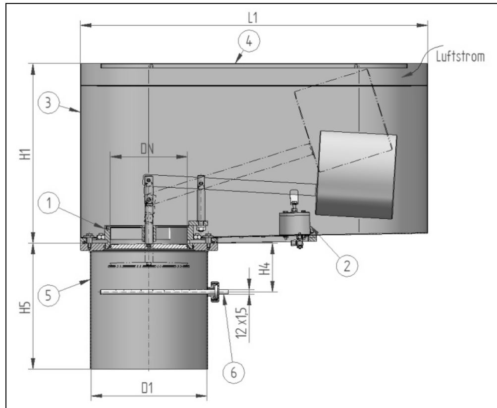
Fig. 4: Tipo 12817 DN 100 – 200 con protección antisalpicada
