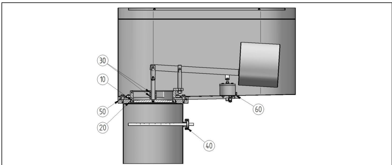
Fig. 7: Typ 12817 DN 100 – 200
