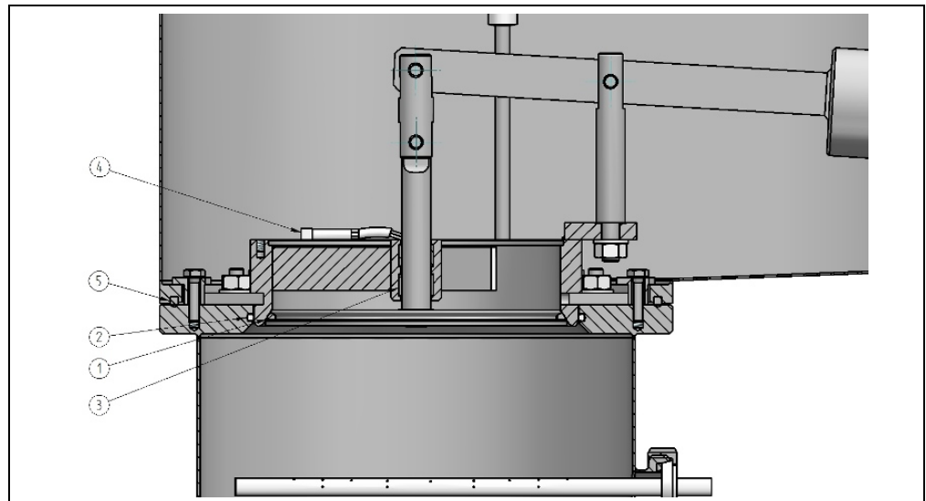
Fig. 5: con cono de acero inoxidable
