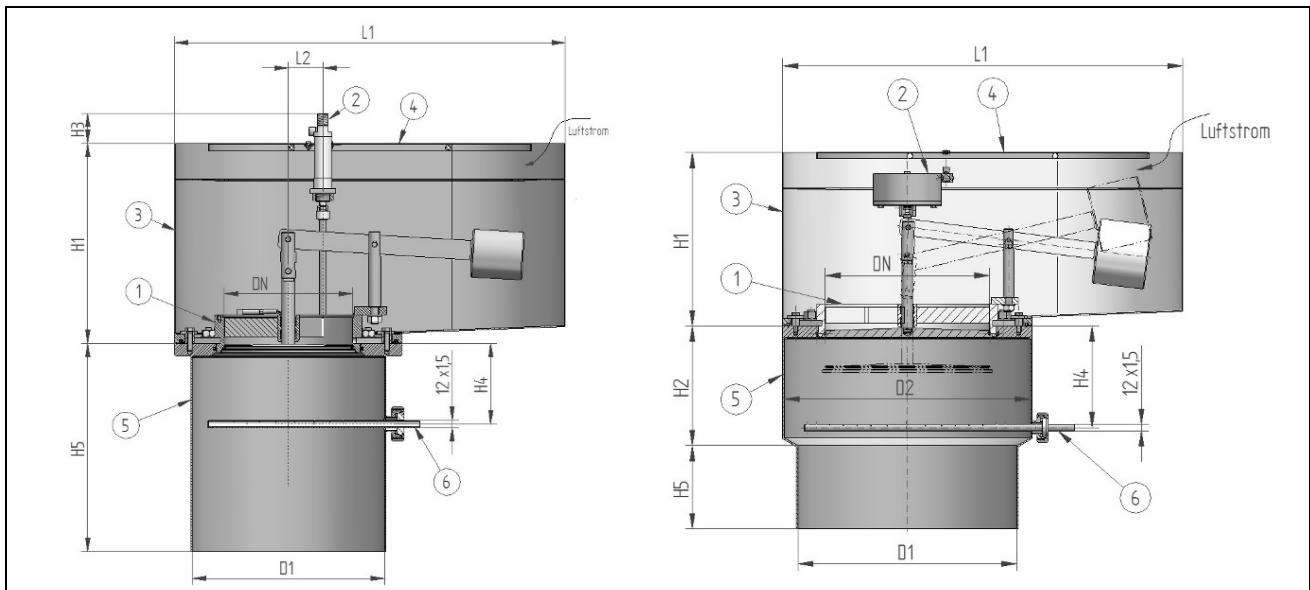
Fig. 3: Tipo 12814 DN 150 - 200 con protección antisalpicada
