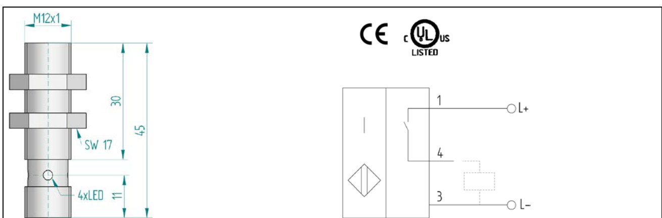
Fig. 9: Dimensiones y esquema de conexión PNP
