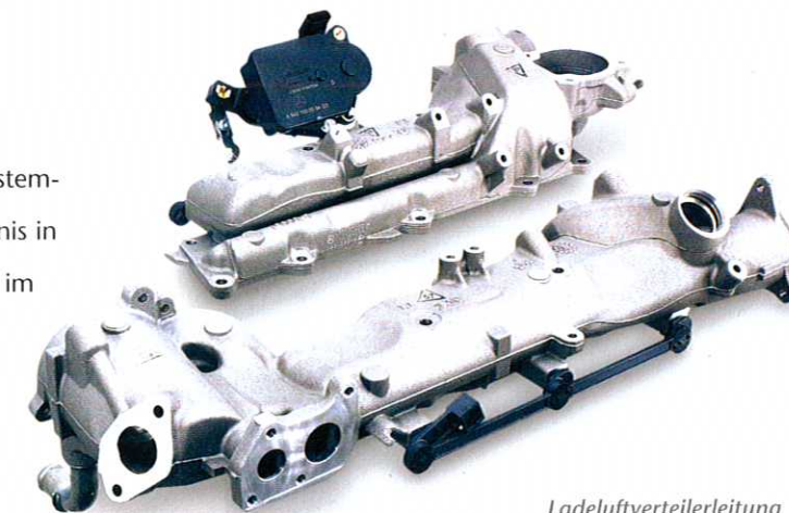
Ladeluftverteilerleitung für Dieselmotor
