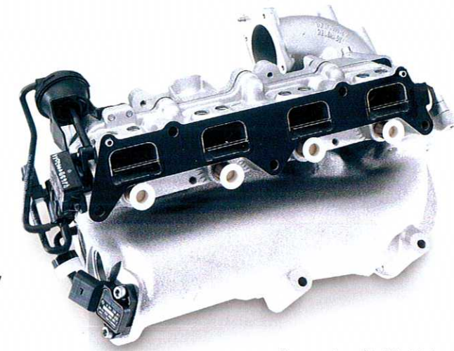
Saugsystem für FSI-Motor komplett montiert
