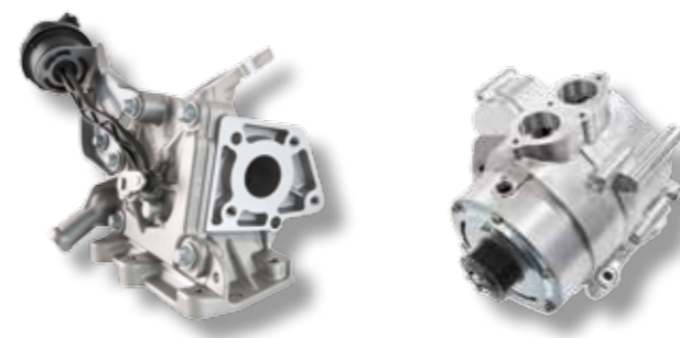
Байпасный клапан LU для 4-цилиндрового дизельного двигателя, используемый с целью сокращения эмиссии вредных веществ. Клапан направляет поступающие выхлопные газы через теплообменник или, в качестве альтернативы, через байпасную линию.
