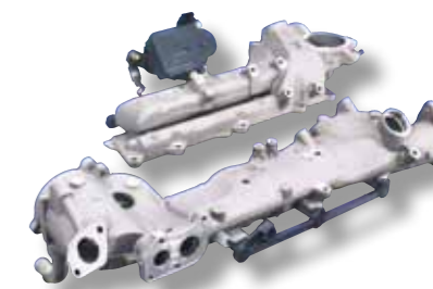
Распределитель нагнетаемого воздуха для 6-ти цилиндрового дизельного двигателя легкового автомобиля, в качестве готовой к монтажу системы.
